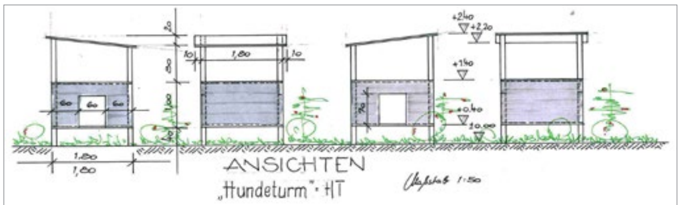
Der zukünftige Hundeturm. Eine gemeinschaftliche Entwicklung und Planung von Mitarbeitern und Vorstand. Zu Papier gebracht und reingezeichnet von Ralf Theissen (Beirat). Wir alle freuen uns auf den Tag, an dem die Hunde ihre Aussichtstürme zum ersten Mal besteigen und genießen können.
